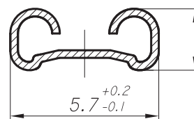
CORTE H-H
