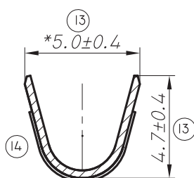
CORTE F-F
