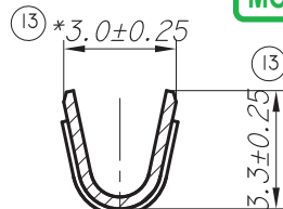
CORTE G-G
